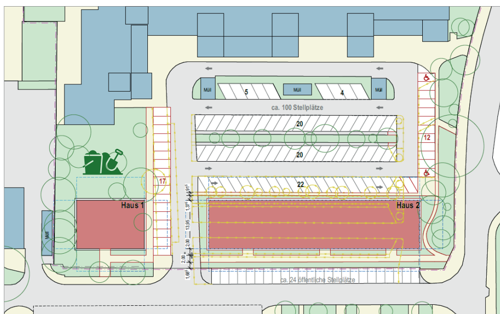
Lageplan, Erschließung/Stellplätze
